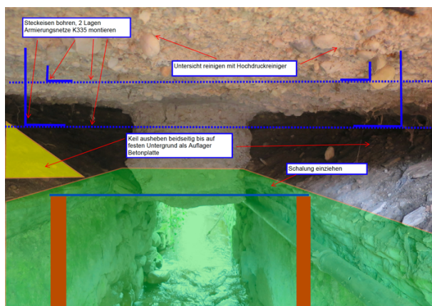
Planung der Sanierung Ländenbachbrücke an der alten Ringwilerstrasse in Ettenhausen
